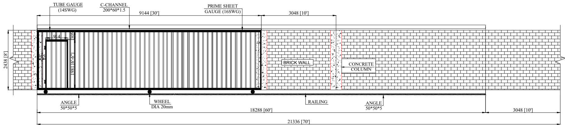
DOOR ELEVATION
